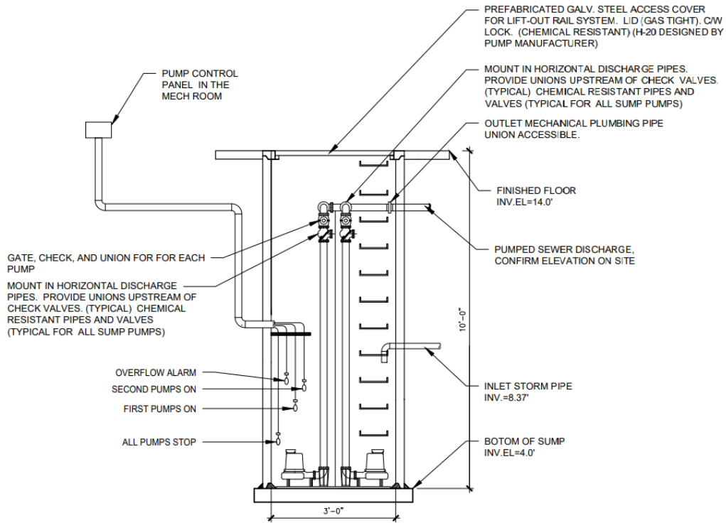
3 STORM PUMP SUMP DETAIL SCALE: N.T.S.
